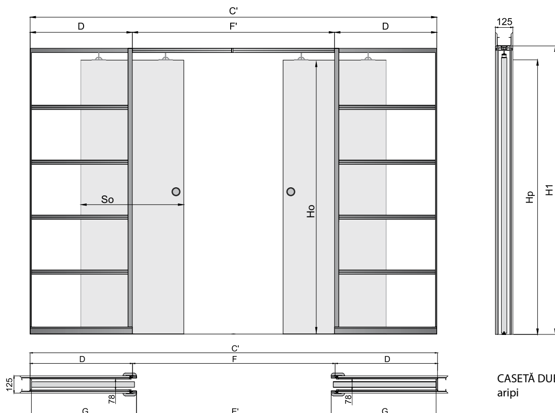
Casetă G/K - sistem glisant de aluminiu dublu
