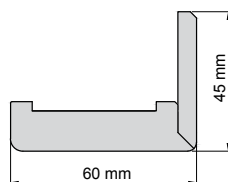
Cornier pentru toc reglabil - lățimea 60 mm
