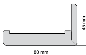
Cornier pentru toc reglabil - lățimea 80 mm
