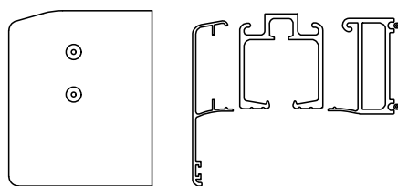
a laguna rendszer elemei
