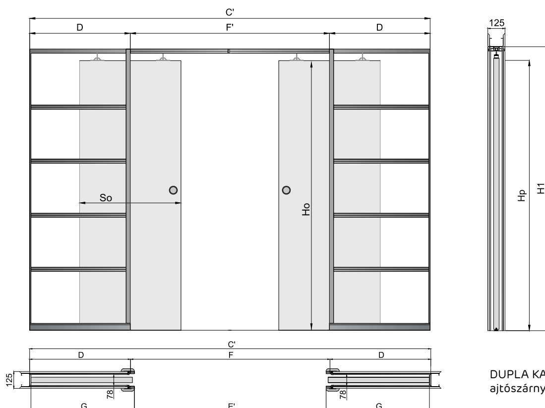
G / K kazetta - dupla alumínium tolóajtó rendszer
