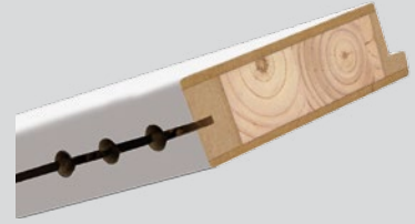
Tömör - masszív KERET szerkezet
