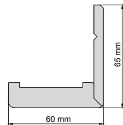
Szélesítő szegőléc a beállítható szélességű ajtótokhoz - szélesség 60 mm
