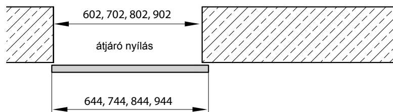
vezető sín
