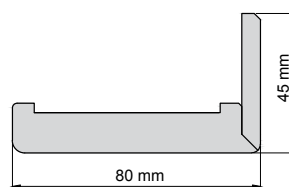
Szegőléc a beállítható szélességű ajtótokhoz - szélesség 80 mm
