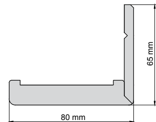
Szélesítő szegőléc a beállítható szélességű ajtótokhoz - szélesség 80 mm
