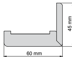
Szegőléc a beállítható szélességű ajtótokhoz - szélesség 60 mm
