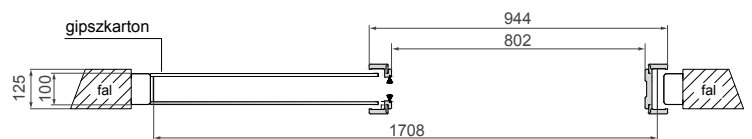
AJTÓTOK 125 TARTOMÁNY - RÖGZÍTETT
