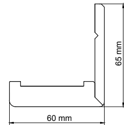
Расширяющий уголок для дверной коробки - ширина 60 мм
