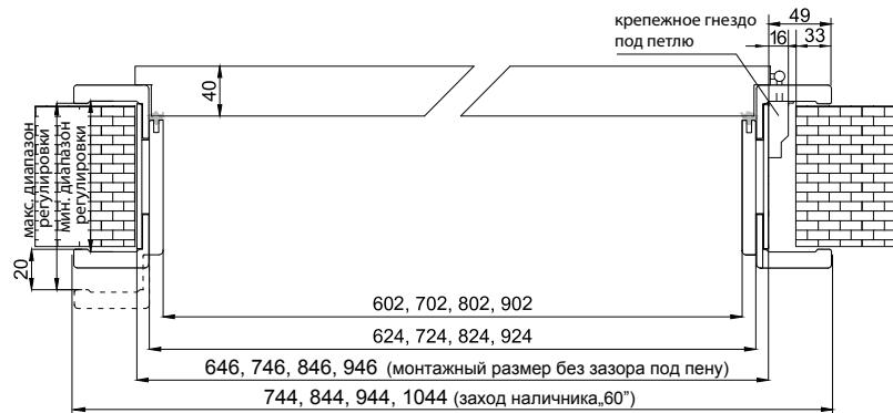
Уголок для регулируемой дверной коробки - ширина 80 мм
