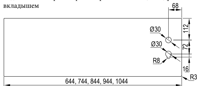
Защитная панель центральная с монтажными отверстиями под замок с заверткой-фиксатором/ ключом/ цилиндровым вкладышем
