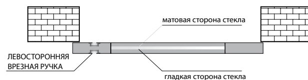
ПРАВОЕ БЕСФАЛЬЦЕВОЕ ДВЕРНОЕ ПОЛОТНО (СДВИГАЕТСЯ ВПРАВО)
