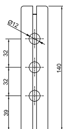
НИЖНЯЯ ЦАРГА РАМЫ ЧЕШСКИЙ СТАНДАРТ
