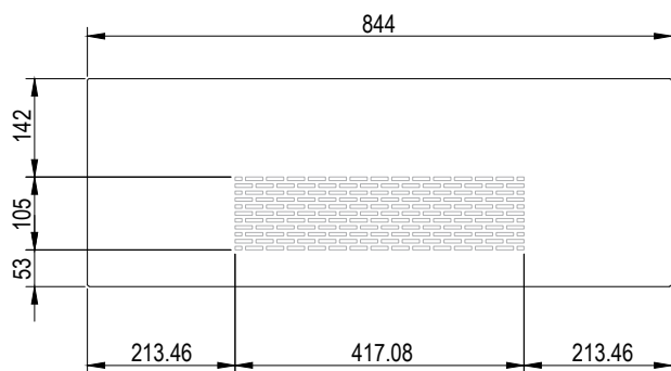
Защитная панель нижняя с вентиляцией, размер для ширины "80"
