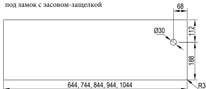
Защитная панель средняя с монтажными отверстиями под замок с засовом-защелкой
