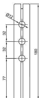
НИЖНЯЯ ЦАРГА РАМЫ
