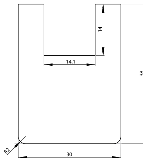
ДЕКОРАТИВНАЯ РЕЙКА (длина 2800)
